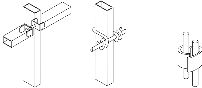
קליפס רשת לרשת חובק רשת לעמוד מחבר "עיוור"
